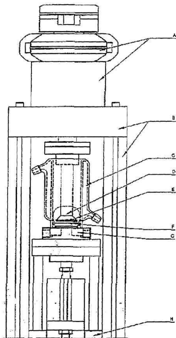
Рисунок 4 – Прибор Б
