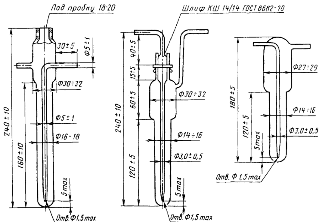
Рис.6. Поглотительные сосуды Все размеры указаны в миллиметрах
