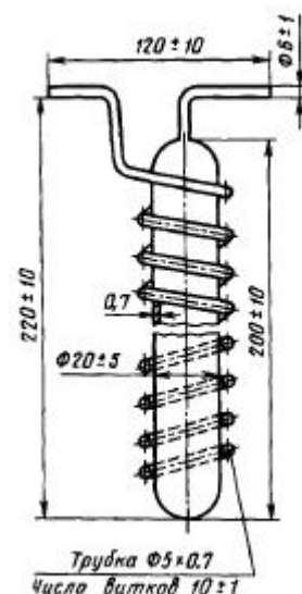
Рис.5. Змеевиковый конденсатор Все размеры указаны в миллиметрах
