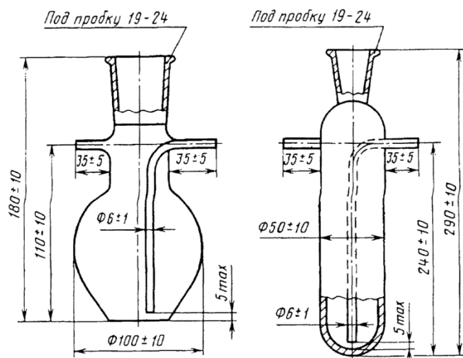
Рис.4. Пробоотборники – испарители Все размеры указаны в миллиметрах
