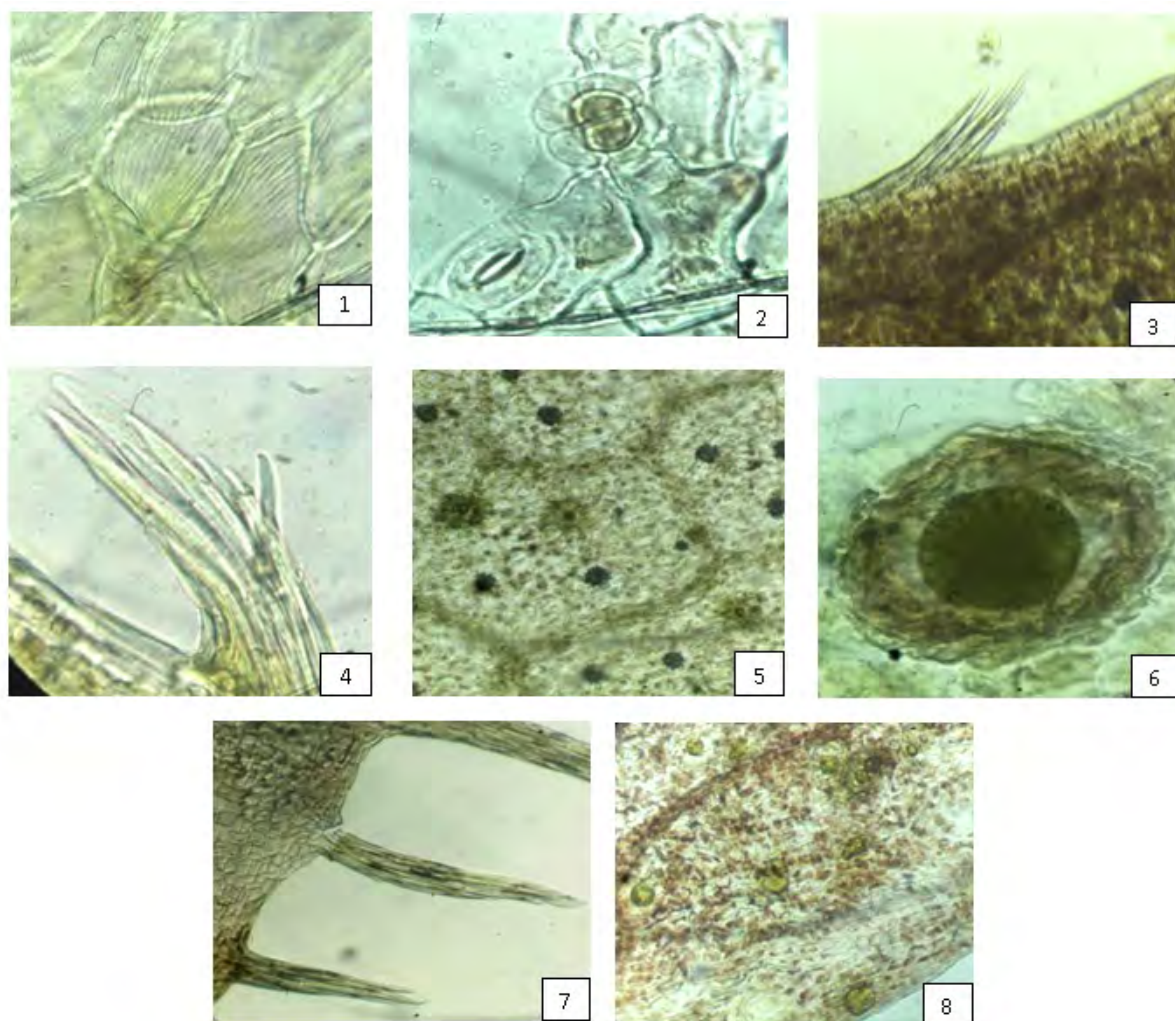
Рис. 1 – Горца перечного трава
